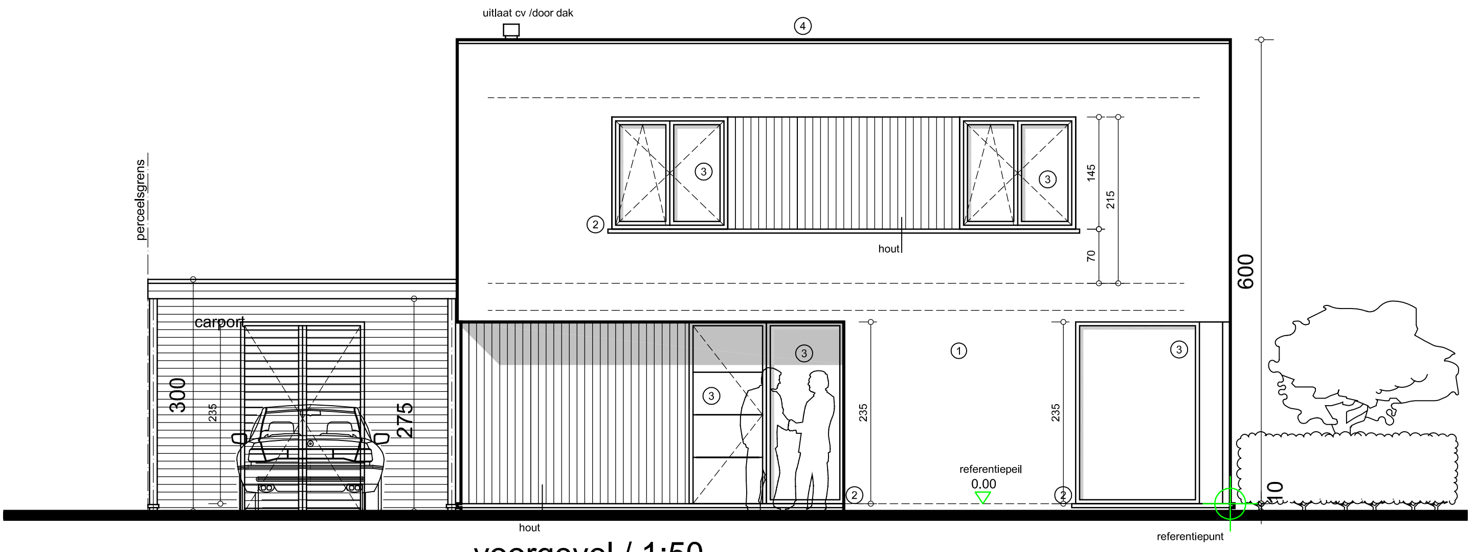
voorgevel / 1:50
